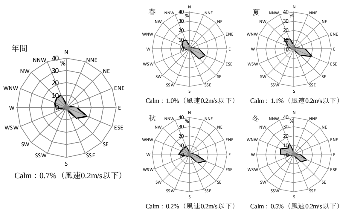
第 3.1-2 図 (2) 風配図 (平成 27 年 : 山口地域気象観測所)
