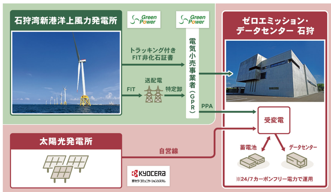
再エネ地産地消事業モデルのスキーム（イメージ）
